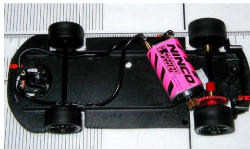
IMAGEN 3. Posición del motor permitida.
